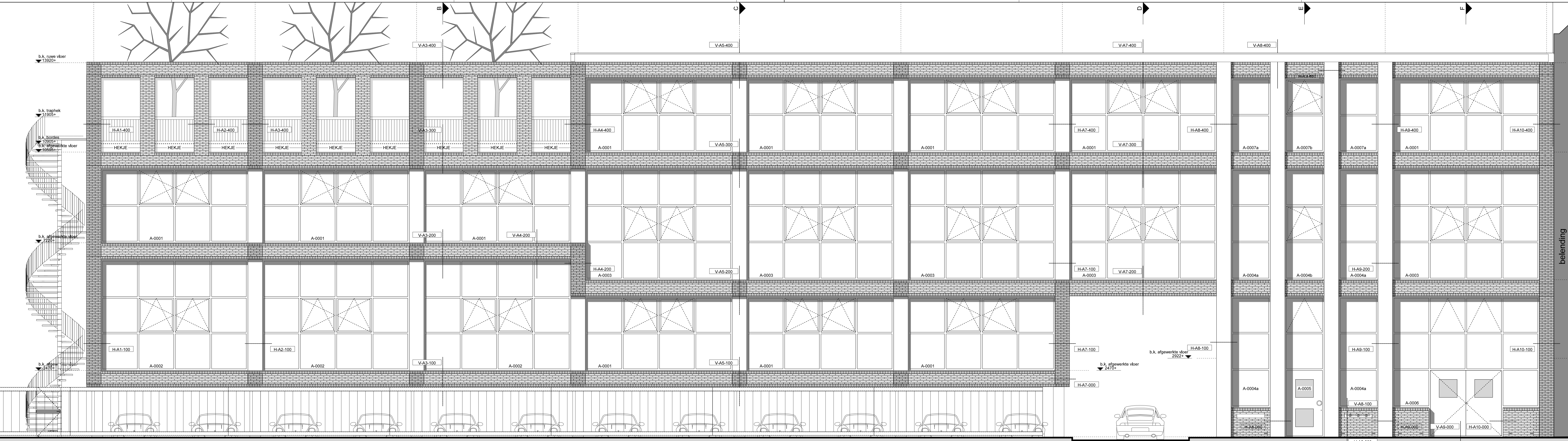
VOORGEVEL AANZICHT WEST
